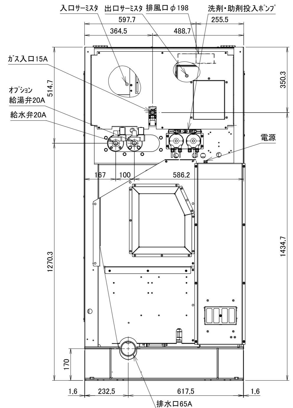
WD6-11JC1外観図
