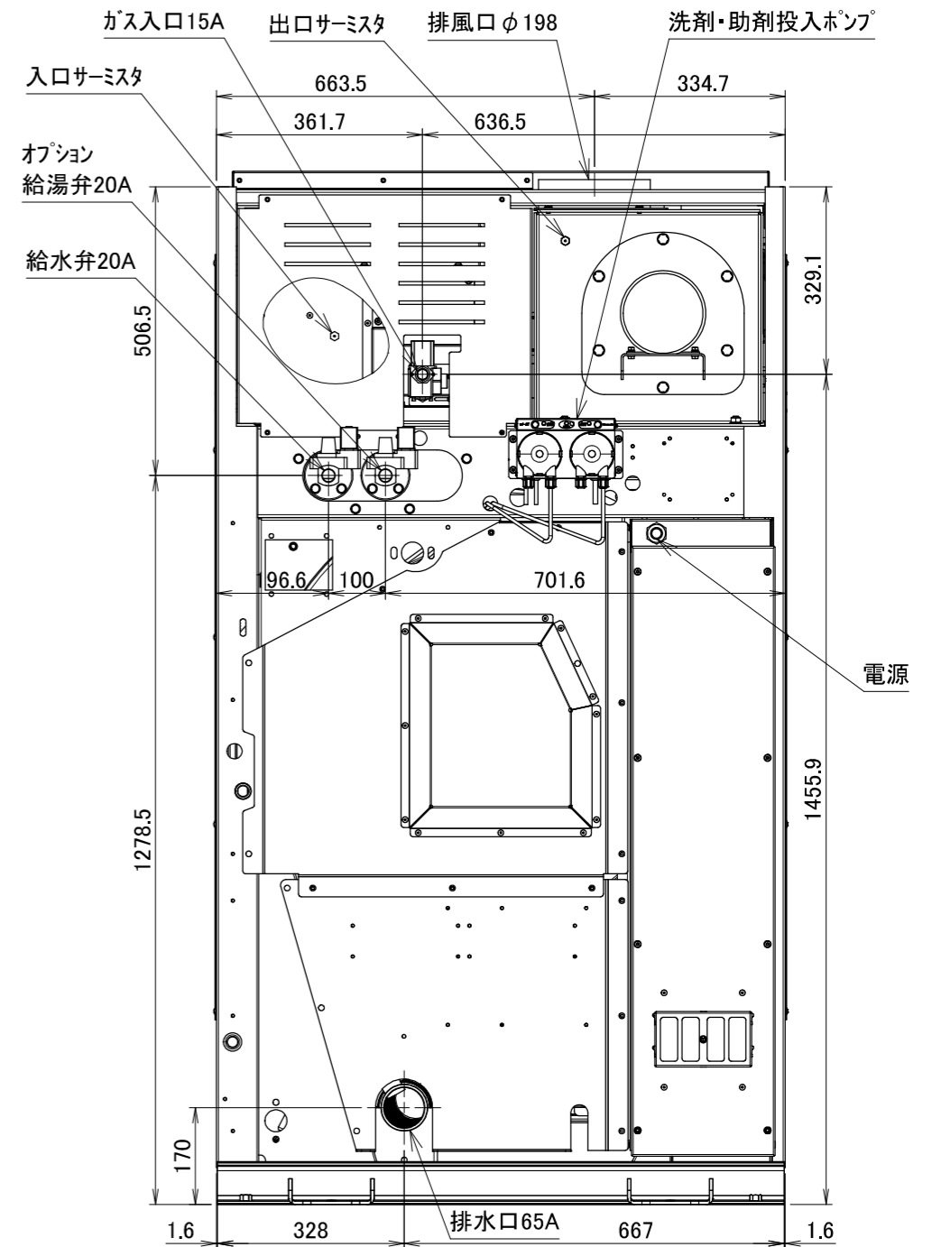
WD6-18JC1 外観図
