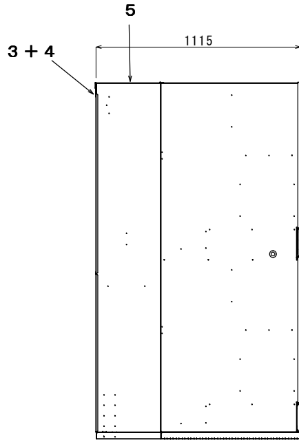
左側面
